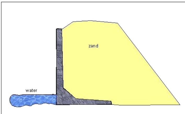
Dwarsdoorsnede ijsvogelwand
